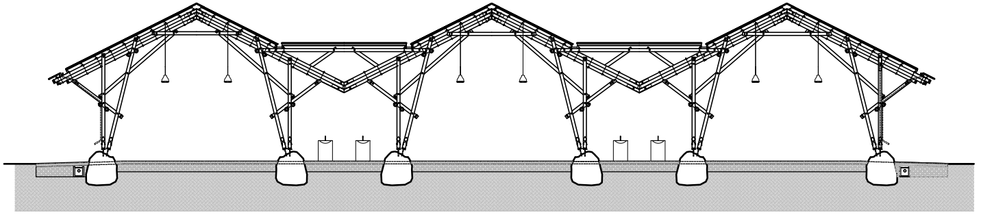
剖面圖一
