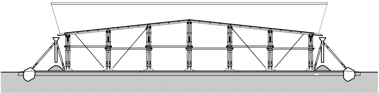
剖面圖四
