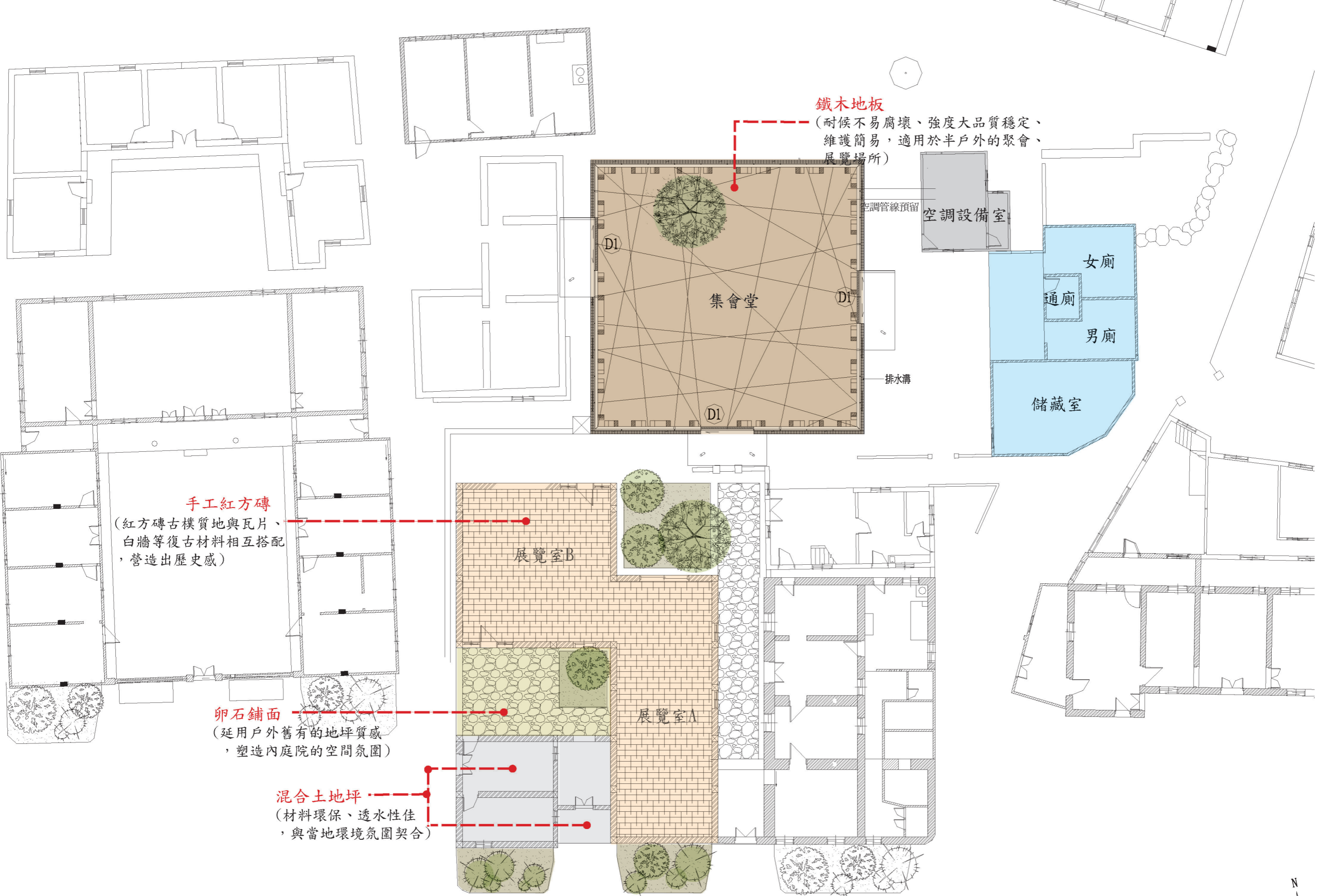
竹北市新瓦屋林姓聚落 展覽室、集會堂平面圖
