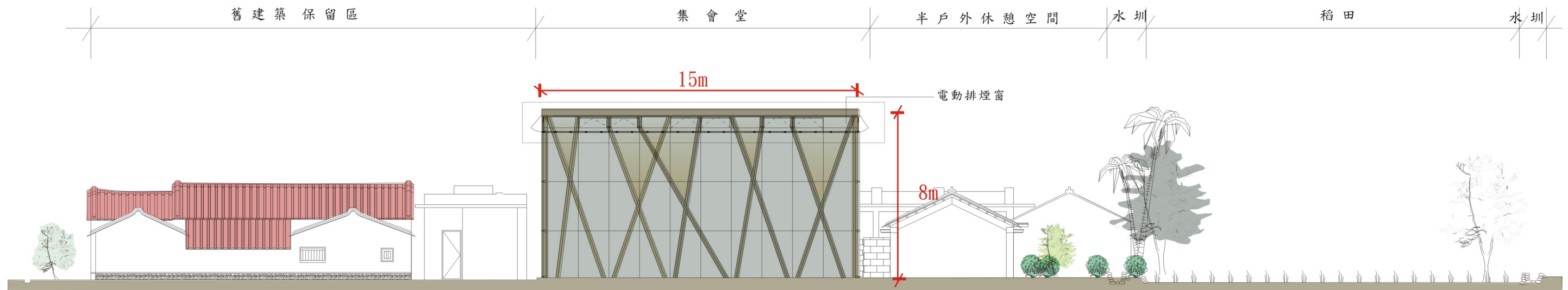
竹北市新瓦屋林姓聚落 展覽室、集會堂立面圖1
