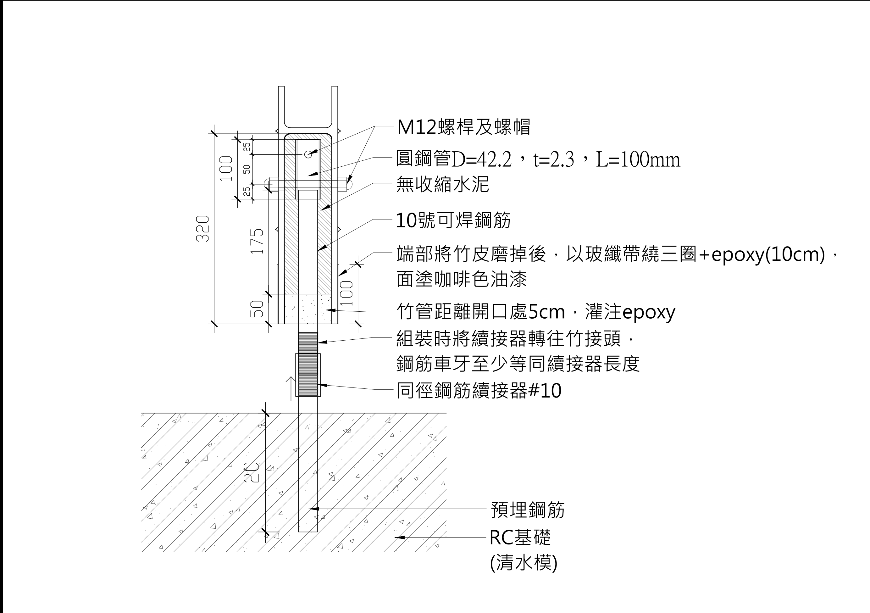
2 接頭A細部 S:1/4(A1) 單位:mm
