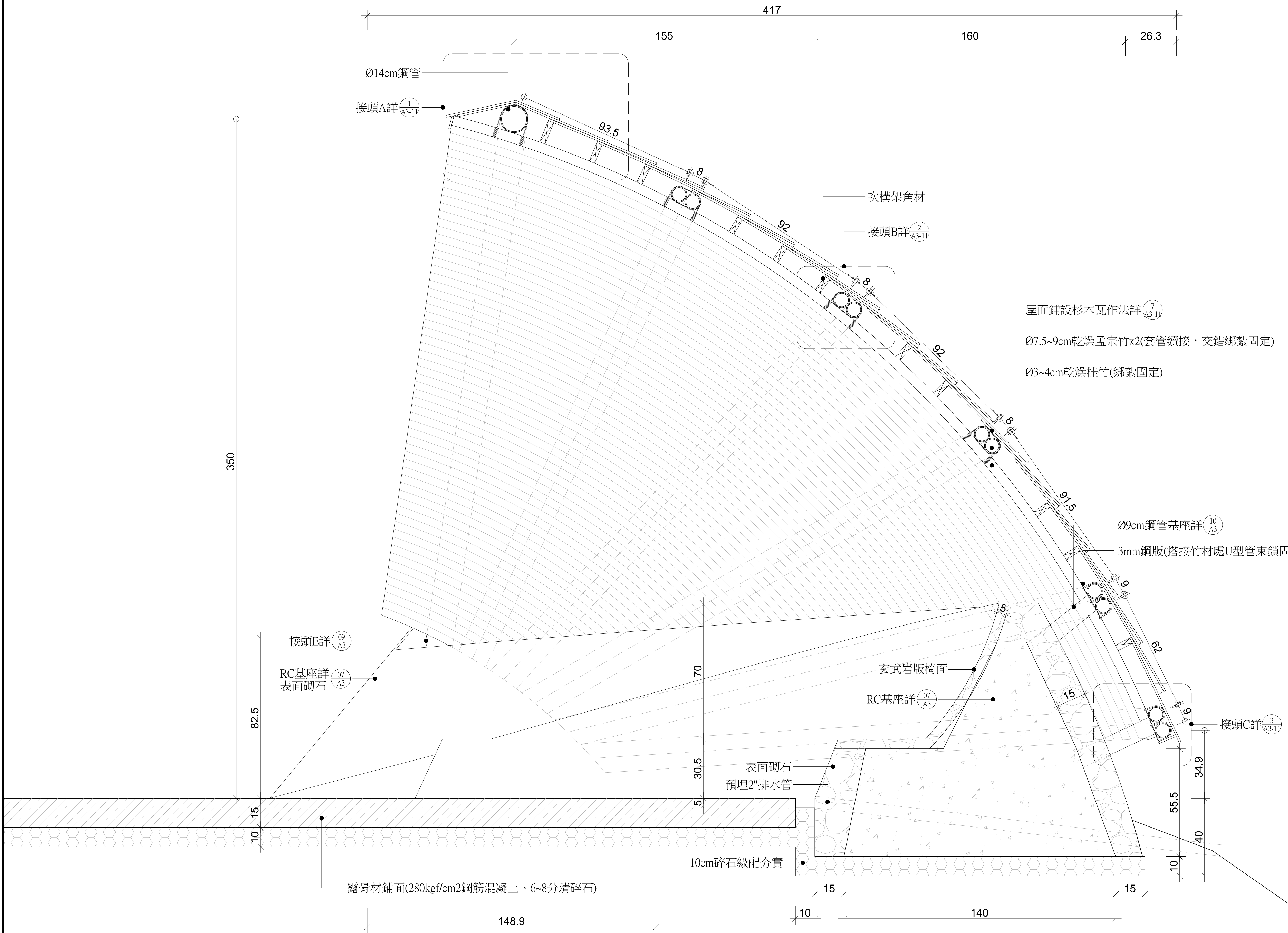
① 橫向剖面圖
