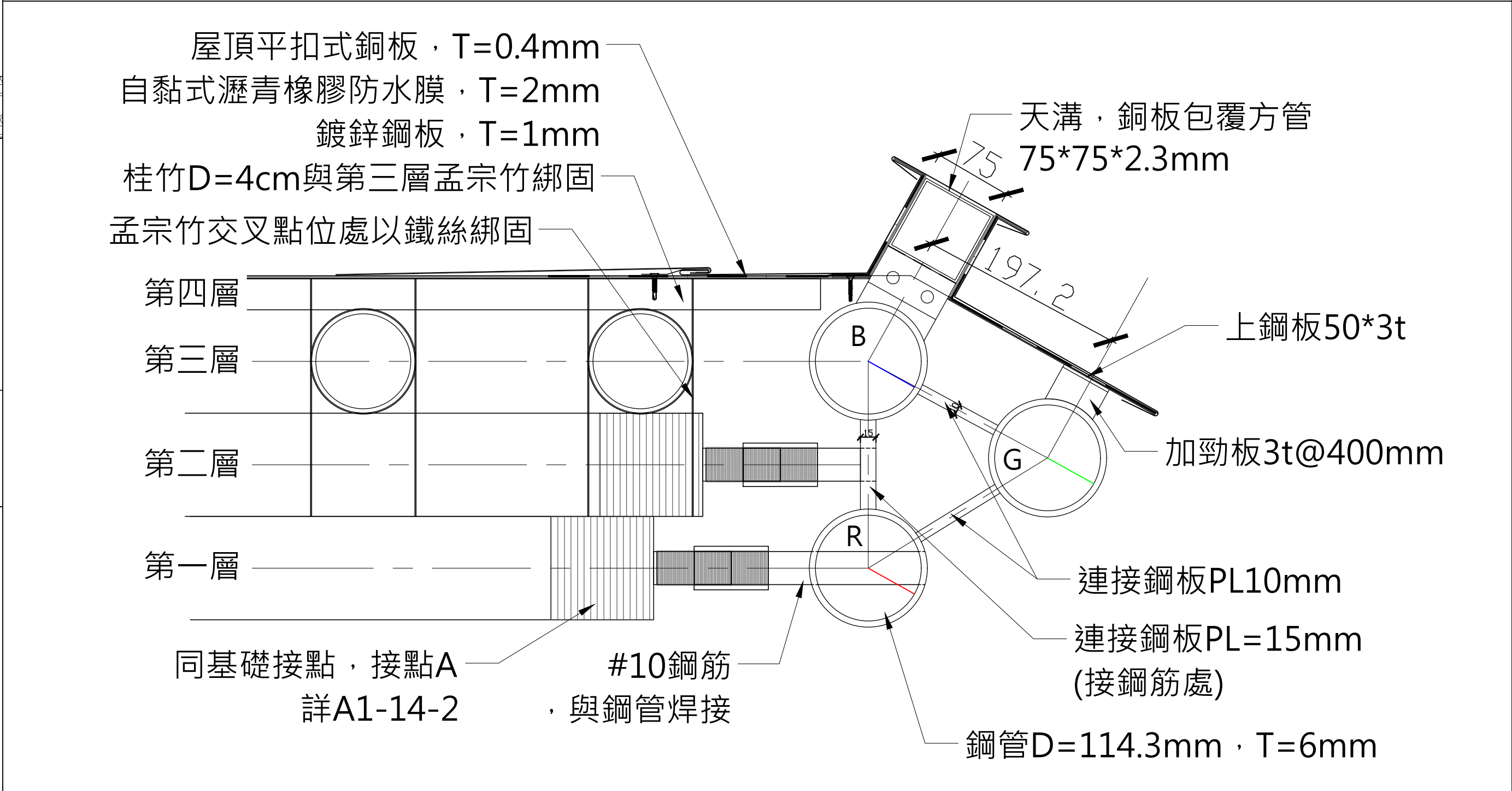
4 接頭C細部 S:1/4(A1) 單位:mm
