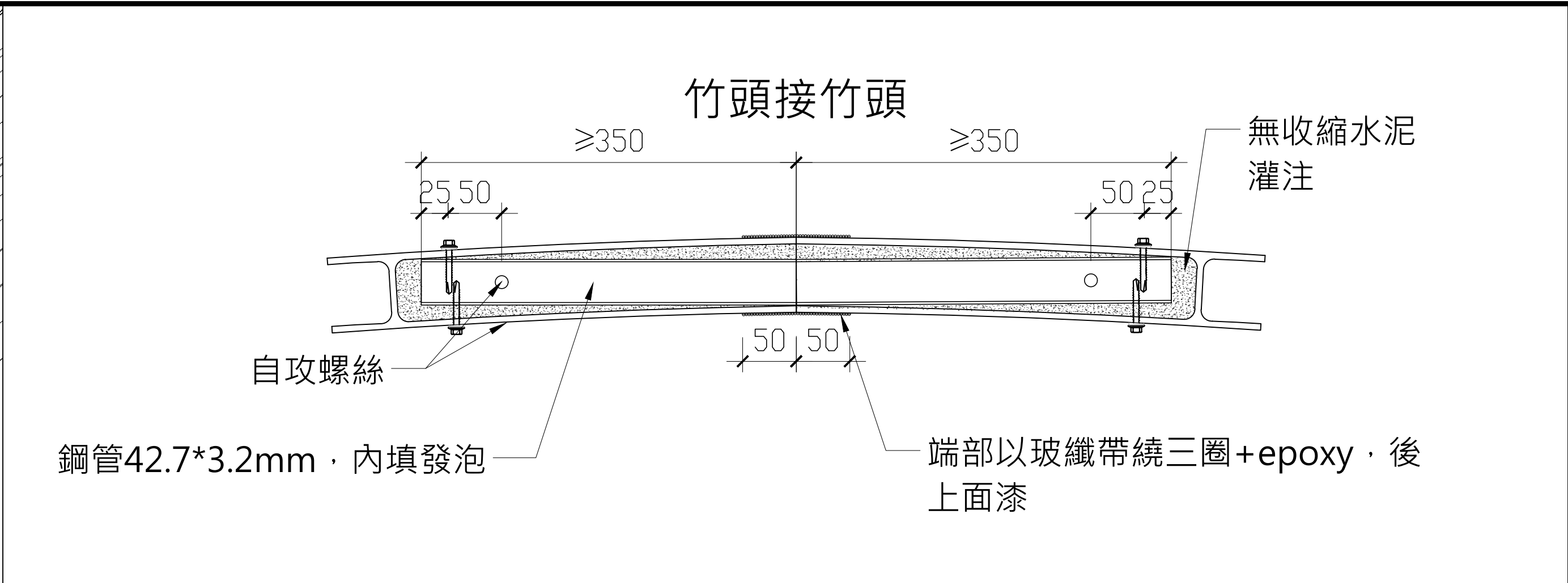
3 接頭B細部 S:1/4(A1) 單位:mm
