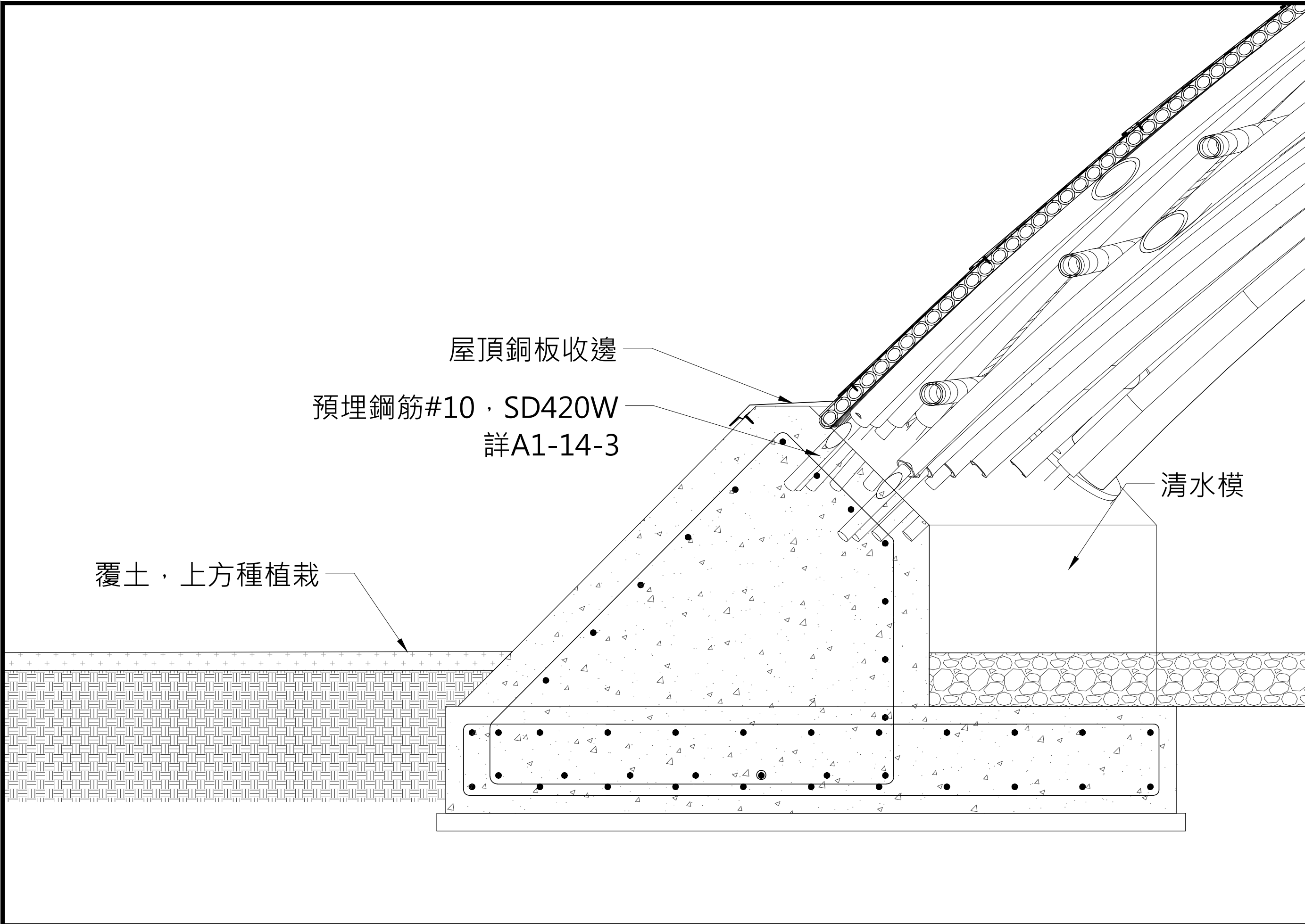
1 基礎細部 S:1/10(A1)
