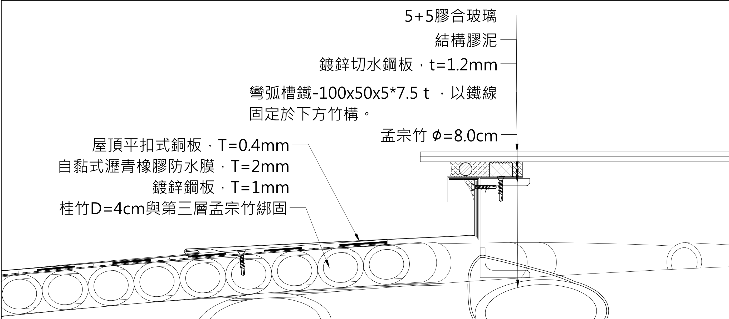
5 接頭D細部 S:1/4(A1)
