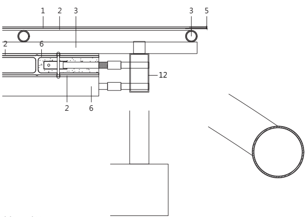
簷口詳圖
