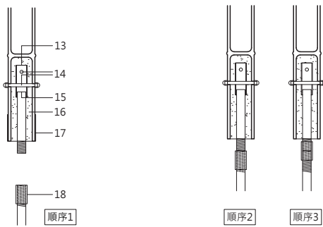
孟宗竹接頭與鋼筋續接器
