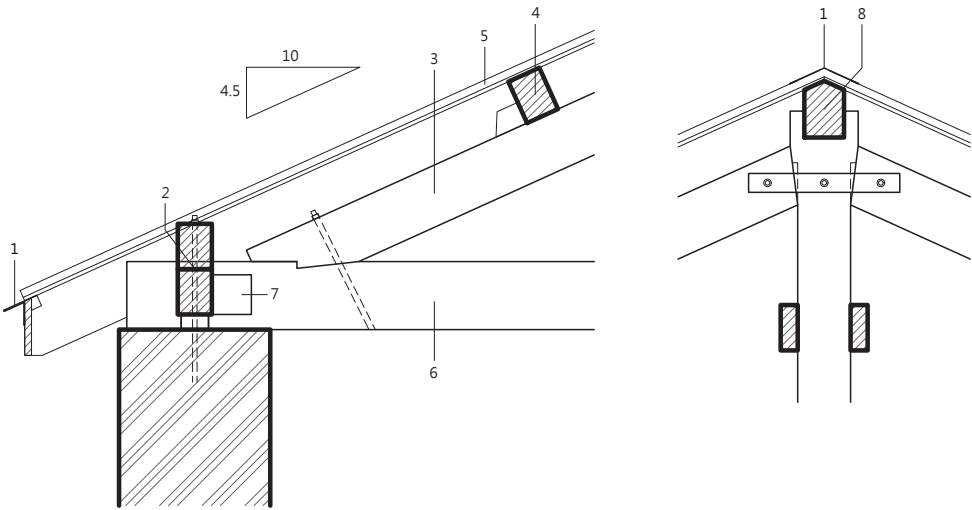
磚造活動中心木屋架構造詳圖
