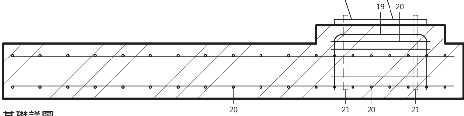
基礎詳圖
