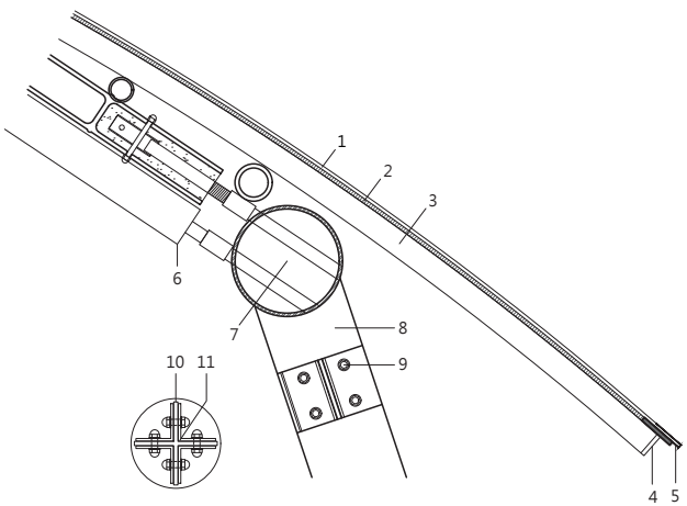
屋面構造詳圖
